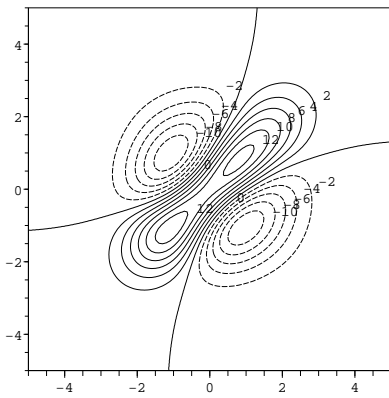
(e) Matrice B
