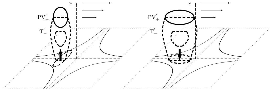
Fig. 3.16: Contribution d'une anomalie de PV au mouvement vertical en dessous. D'après Arbogast (1998)
