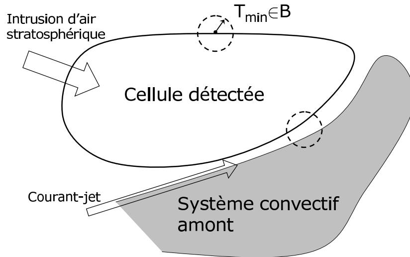
Fig. 1.15: Calcul de la distribution du minimum de température dans un voisinage du contour d'une cellule afin de déterminer le quantile de nuages environnant, et de sélectionner les intrusions sèches. B désigne la boule utilisée pour le calcul de la température minimale T_{\min} dans un voisinage du contour.
