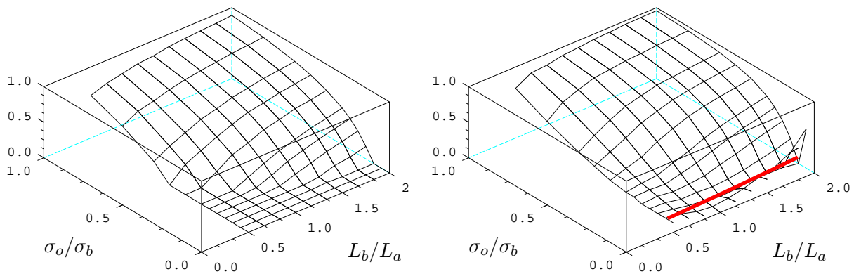
(c) Mesure d'erreur \mathcal{E}_{\text{dep}}
