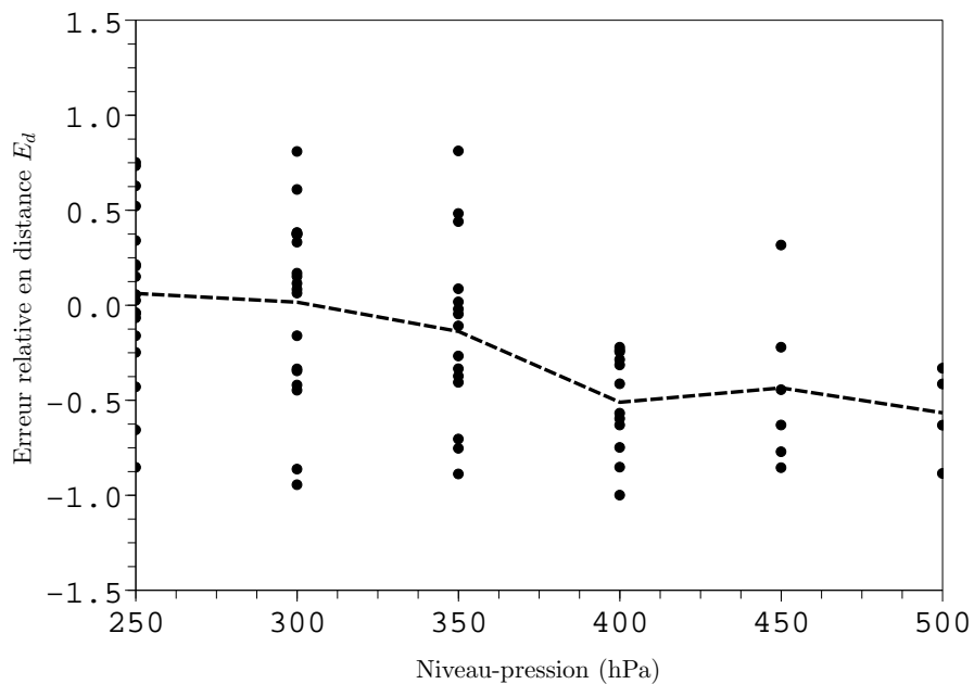
(b) Erreur relative de déplacement
