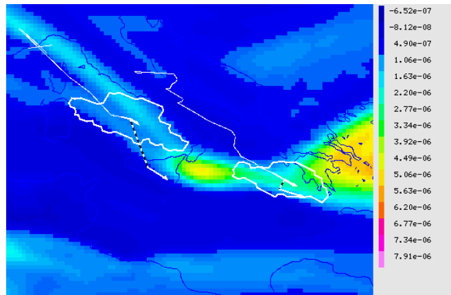
Fig. 3.20: Tourbillon potentiel à 300 hPa (ébauche opérationnelle ARPEGE) et cellules du traitement Antidote appliqué sur les images modèle (en blanc). Situation au 29 Avril 2007 à 00 TU.
