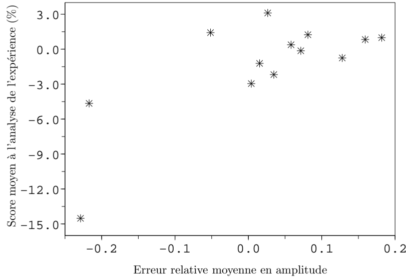
Fig. 4.28: Tracé du score à l'analyse (moyenné sur les trois échéances 24, 48 et 72 heures) pour chaque expérience en fonction de l'erreur d'amplitude (moyennée sur les différentes cellules et niveaux).
