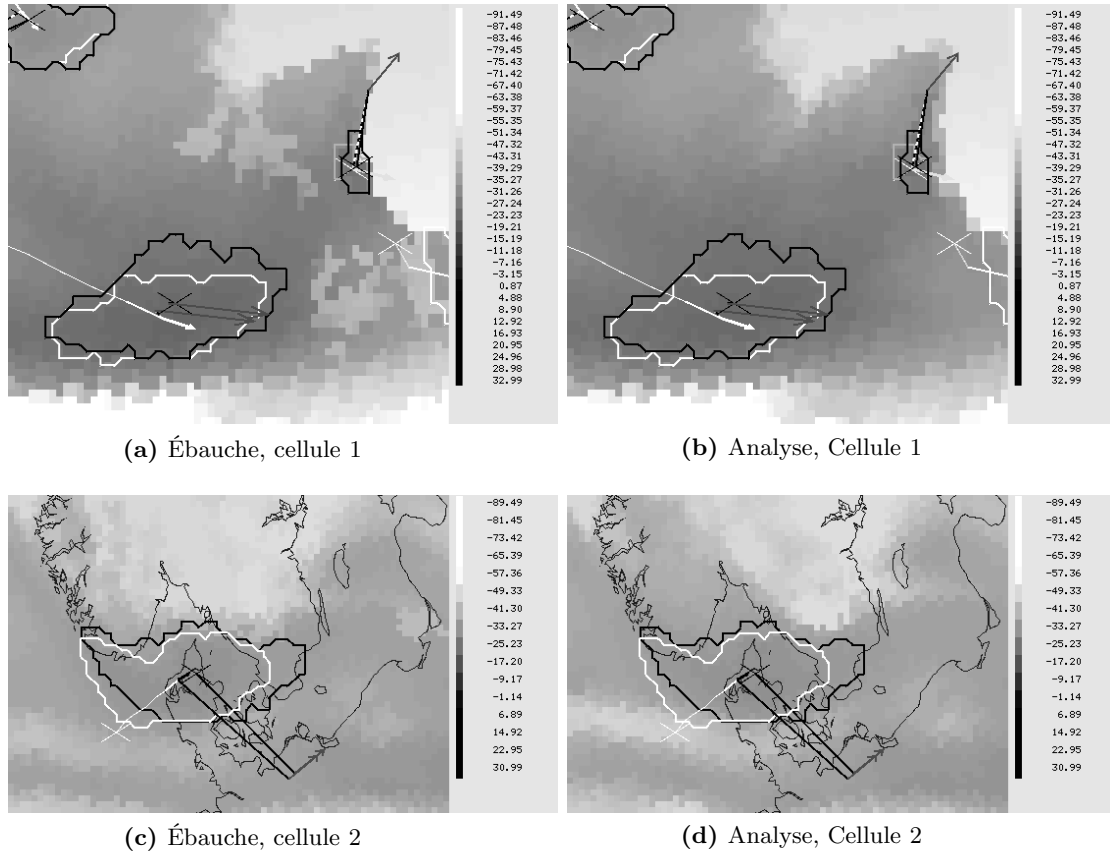
Fig. 4.24: Images vapeur d'eau MSG au 20 Mai 2006 00 TU superposées au traitement d'images Antidote (contours et trajectoires des cellules satellite en noir, modèle en blanc). Ebauches à gauche; analyses issues de l'assimilation des pseudo-observations de déplacement en tourbillon potentiel à droite.
