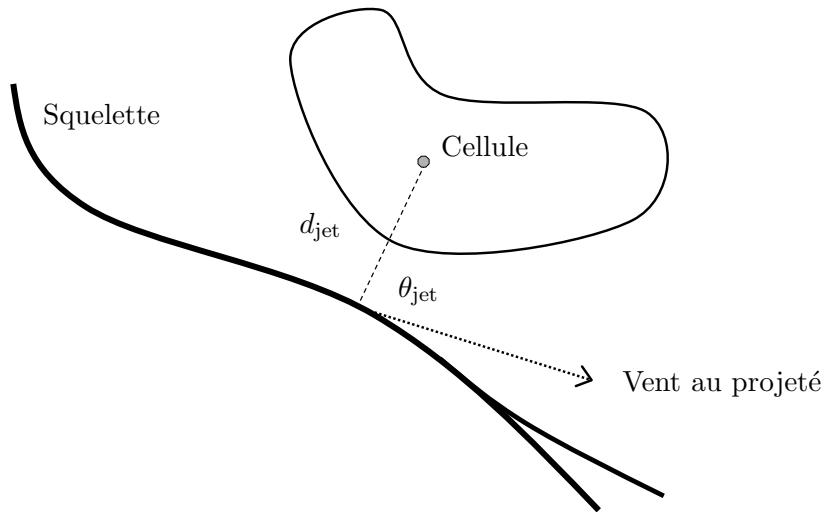
Fig. 1.24: Calcul de la projection sur le squelette du courant-jet.
