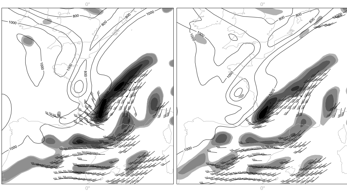
(c) Prévission REF du 01 octobre à 12 TU pour le 03 octobre à 06 TU
