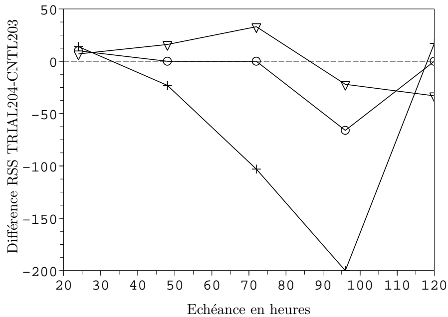
Fig. 5.4: Différence TRIAL204-CNTL203 pour les scores d'habileté relatifs (RSS) en intensification (signes +), en dissipation (triangles) et en tendance (cercles).
