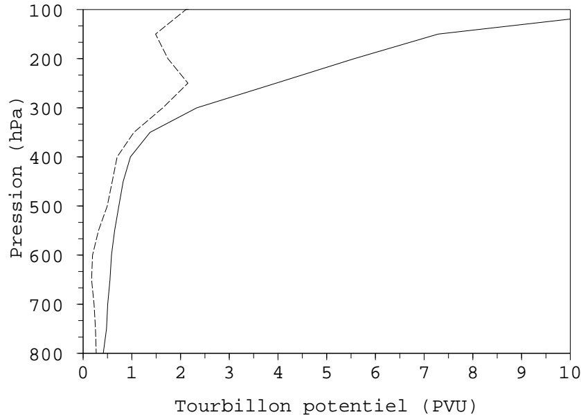
Fig. 3.5: Profil des valeurs moyennes de tourbillon potentiel \overline{PV_j} (traits pleins) et des écarts-types en tourbillon potentiel (traits tiretés).
