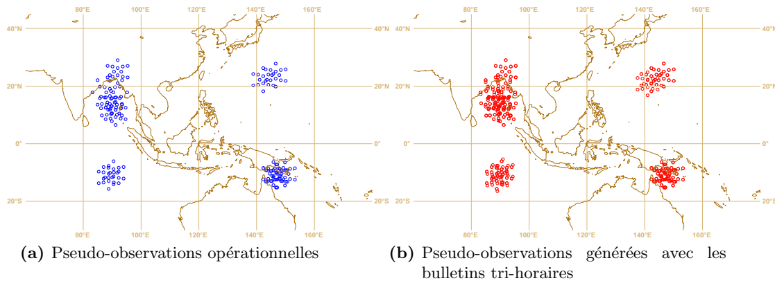
Fig. 5.2: Pseudo-observations de cyclones tropicaux sur la période 20071012-20071016 (dont le cyclone Sidr).
