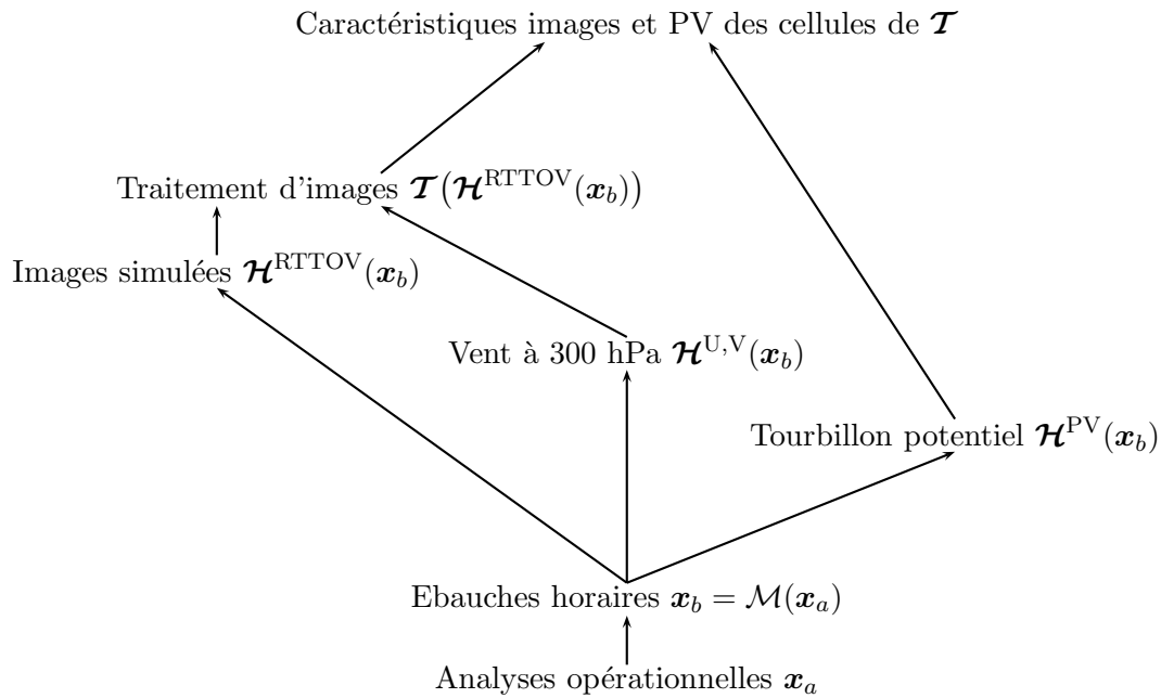
Fig. 3.1: Application des différents opérateurs d'observation et de traitement d'image pour l'étude de la relation PV-WV.
