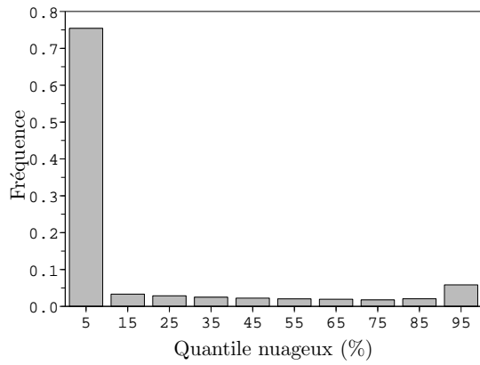
(a) Toutes cellules de durée supérieure à trois heures, T_{\text{cld}} = -54 \text{ }^\circ\text{C}
