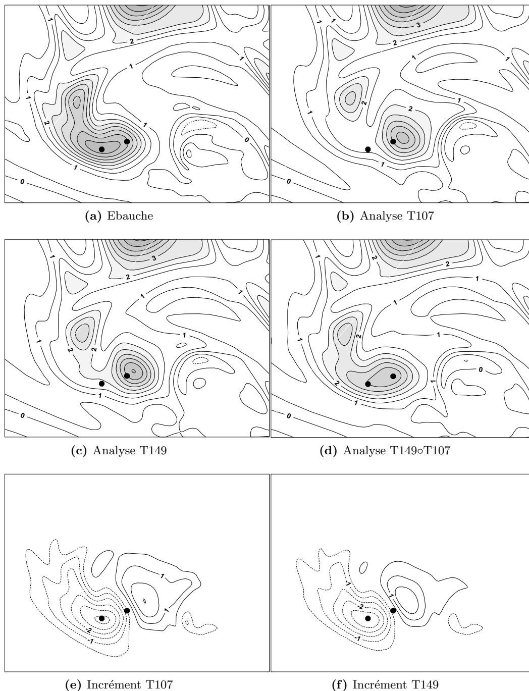
Fig. 4.16: Assimilation à T107, T149 et T149◦T107, cellule 1. Expérience d'assimilation ARPEGE de pseudo-observations de déplacement à la date du 20/05/2006 00 TU au niveau 350 hPa. Champs de tourbillon potentiel. Intervalle de contour 0.5 PVU, contour 0 PVU en traits gras. Niveaux de gris à partir de 2 PVU. Les disques représentent les pseudo-observations introduites pour les cellules détectées, appariées, et conduisant à la génération d'observations. \sigma_o = 0.1 \cdot \tilde{\sigma}_b .
