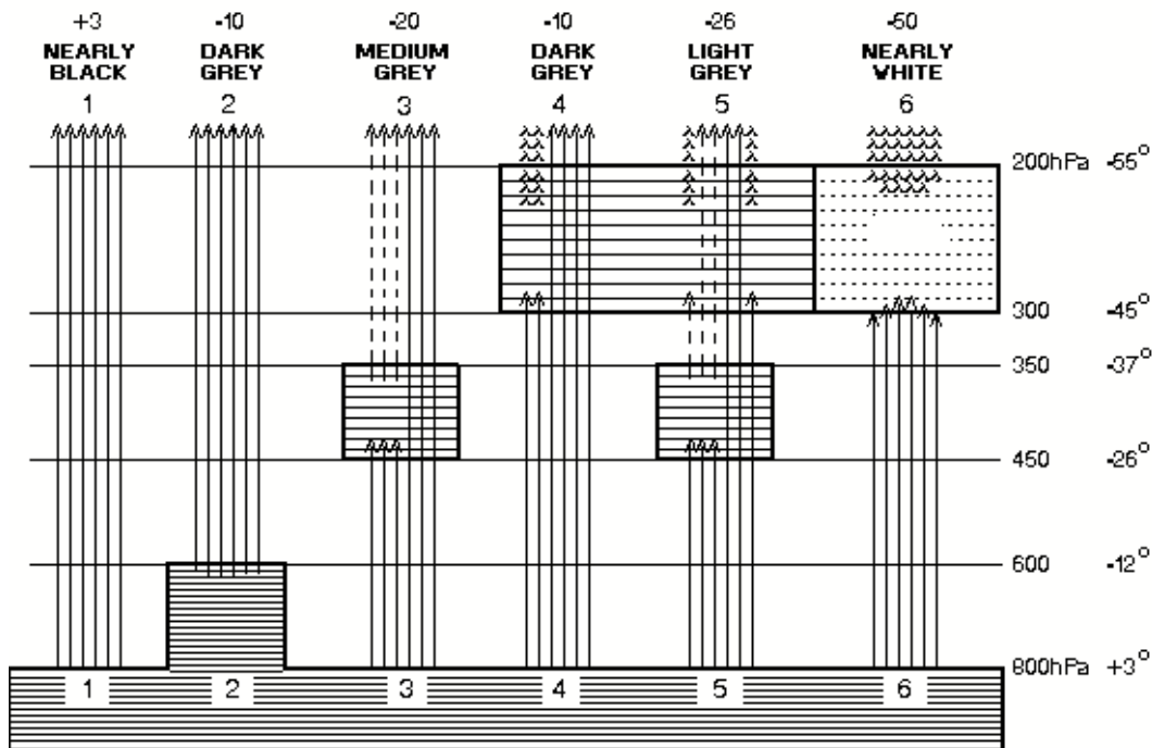
Fig. 1.7: Influence des couches d'humidité sur le canal vapeur d'eau 6.7 \mu\text{m} , d'après Weldon et Holmes (1991).
