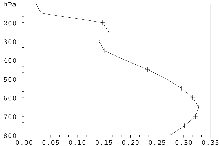
Fig. 3.18: Coefficient de corrélation pour les régressions linéaires entre la vitesse verticale moyennée sur la surface des cellules à un niveau isobare et la variation Lagrangienne de température de brillance maximale de ces mêmes cellules détectées par Antidote (1570 cas).
