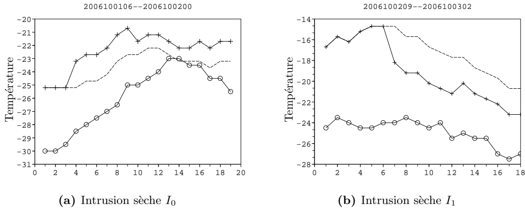
Fig. 6.7: Températures de brillance comparées des intrusions modèle et satellite pour I_0 et I_1 . Cercles : température de la cellule satellite ; croix : température de la cellule modèle ; pointillés : température modèle corrigée des sauts de température aux réseau d'assimilation.
