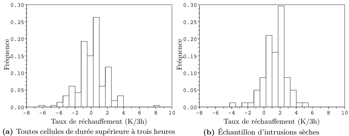
Fig. 1.12: Distributions des réchauffements maximums le long des trajectoires dans l'échantillon d'apprentissage supervisé.
