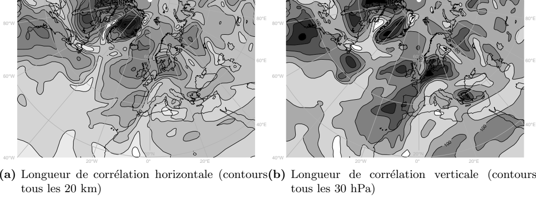
Fig. 2.13: Diagnostics de longueurs de corrélation dans l'espace tourbillon potentiel pour l'analyse ARPEGE au 01 décembre 2006 00TU. Estimation par tirage statistique d'éléments de perturbations de covariance B ( N_{\text{BGVECS}} = 625 correspondant à une précision relative de \simeq \frac{1}{50} ). Niveau 21 du modèle (environ 300 hPa)
