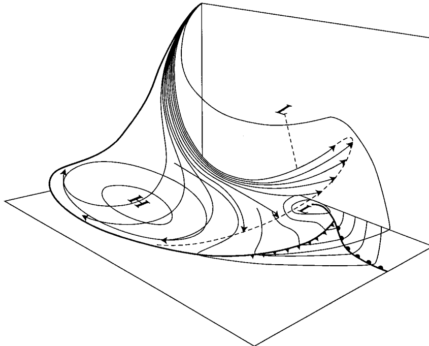
Fig. 1.8: Représentation tridimensionnelle d'une intrusion sèche; figure issue de Browning (1997). Les flèches indiquent les trajectoires sur des surface isentropes des parcelles d'air originaires de la tropopause. Elles arrivent à proximité du sol dans la partie gauche du schéma mais pas dans la partie droite où elles se superposent aux fronts de surface (Browning 1997).
