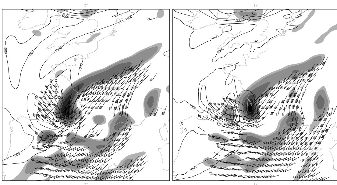
(c) 2006100206, prévision ARPEGE à 24 heures
