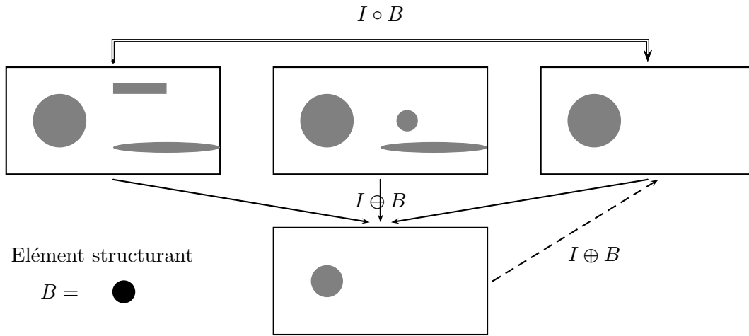
Fig. 1.18: Opérations morphologiques sur des images binaires
