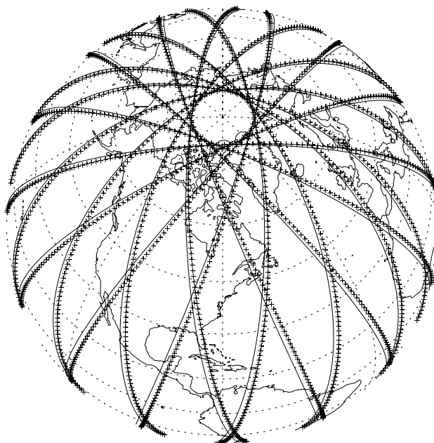
Fig. 6.13: Mesures MLS (croix) le long de l'orbite du satellite Aura (traits continus) pendant une période de 24 heures.
