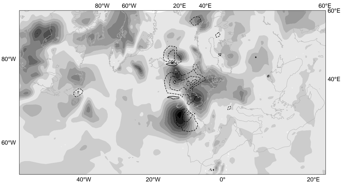
Fig. 4.25: Erreur quadratique de l'ébauche : niveaux de gris tous les 1 hPa, à partir de 1 hPa. Différences entre erreurs quadratiques de la prévision issue de l'analyse des pseudo-observations et de la prévision issue de l'ébauche : contour tous les 1 hPa, positive (dégradation) en traits tiretés, négative (amélioration) en traits pleins.
