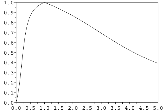
Fig. 4.13: Filtrage spatial \mathcal{F} appliqué à l'erreur de position.
