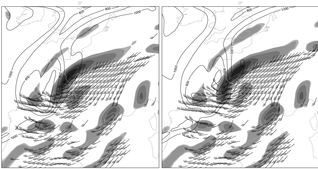
(a) Prévission REF du 01 octobre à 06 TU pour le 03 octobre à 06 TU
