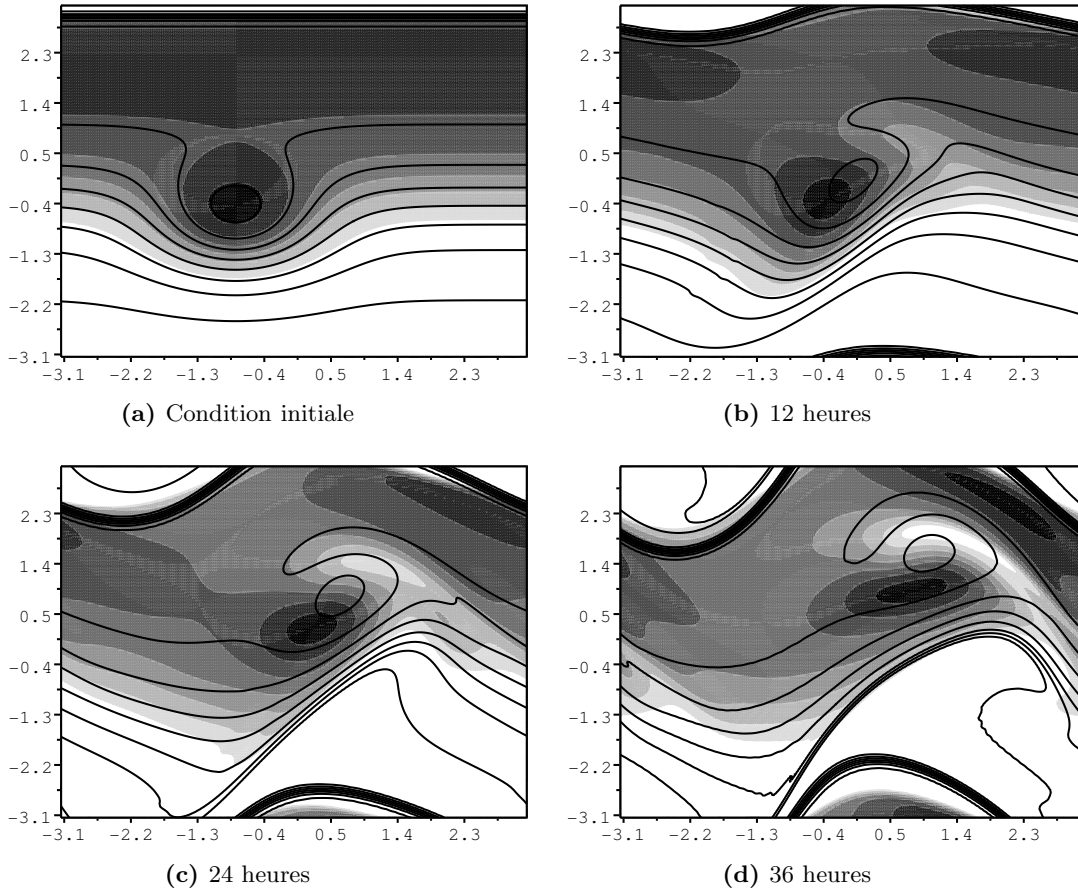
Fig. 3.15: Température de brillance simulée T_{BB} dans le canal vapeur d'eau (niveaux de gris). Les contours en traits pleins délimitent l'anomalie de tropopause \delta_z .
