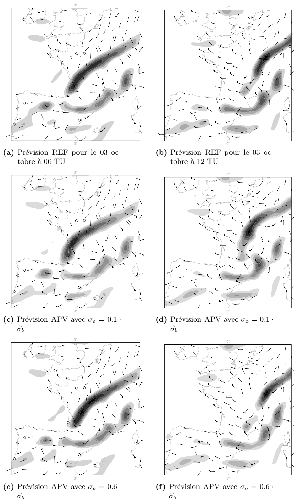
Fig. 6.9: Observations en vent à 10 mètres issues des stations sol (barbules) comparées au tourbillon relatif à 850 hPa (intervalle de gris 5 \cdot 10^{-5} \text{ s}^{-1} ). En haut : prévision opérationnelle; au milieu et en bas prévision avec assimilation des pseudo-observations de PV pour différents \sigma_o .
