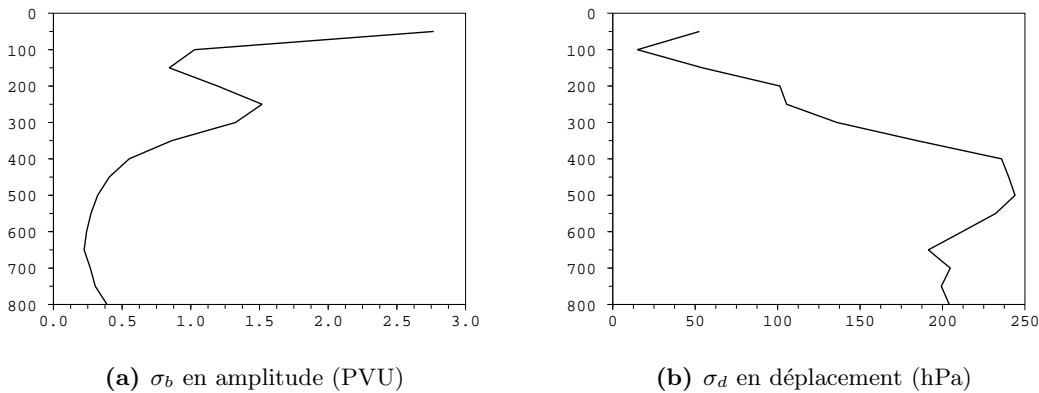
Fig. 2.5: Ecarts-types d'erreurs d'ébauche dans les espaces amplitude et position.
