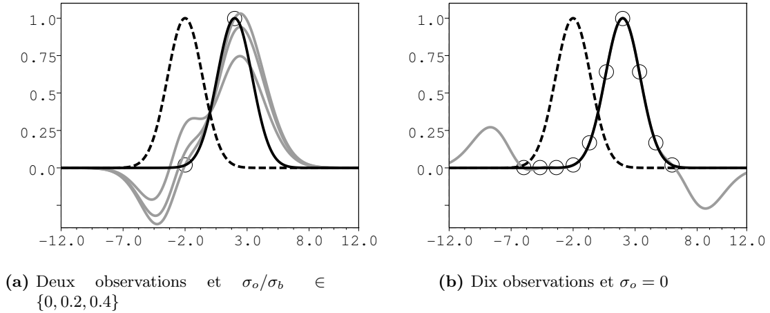
Fig. 4.4: Analyses obtenues pour divers rapports entre écarts-types d'observations et d'erreur d'ébauche. Cas où L_b > L_a . Légende identique à celle de la figure 4.3.
