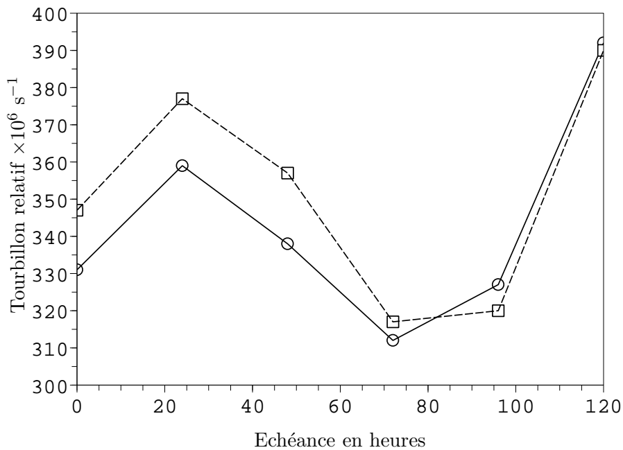
Fig. 5.5: Tourbillon relatif moyen aux centres des cyclones tropicaux dans les deux expériences. CNTL203 en traits pleins et cercles, TRIAL204 en traits tiretés et carrés.
