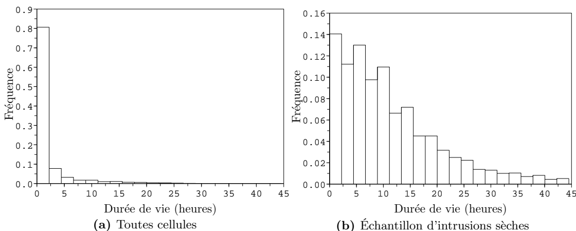
Fig. 1.11: Distributions des durées de vie dans l'échantillon d'apprentissage.
