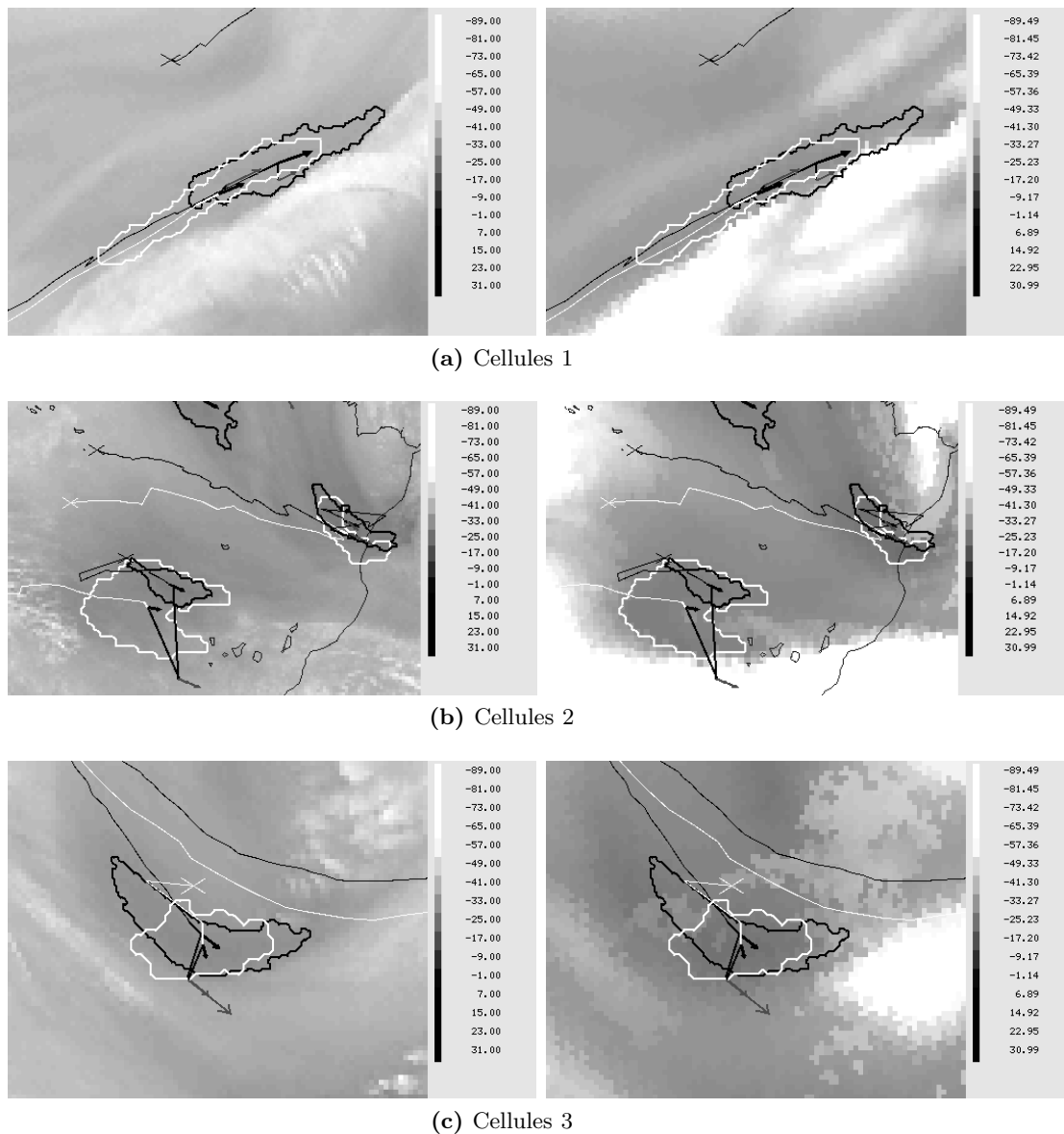
Fig. 4.11: Images vapeur d'eau MSG au 07 Novembre 2006 12 TU (satellites à droite, issues de RTTOV à gauche) superposées au traitement d'images Antidote (contours et trajectoires des cellules satellite en noir, modèle en blanc).
