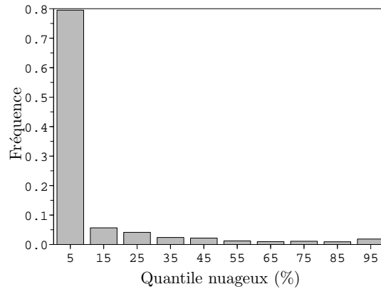
(d) Intrusions sèches, T_{\text{cld}} = -50 \text{ }^\circ\text{C}
