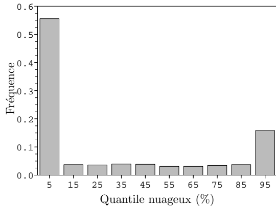
(c) Toutes cellules de durée supérieure à trois heures, T_{\text{cld}} = -50 \text{ }^\circ\text{C}
