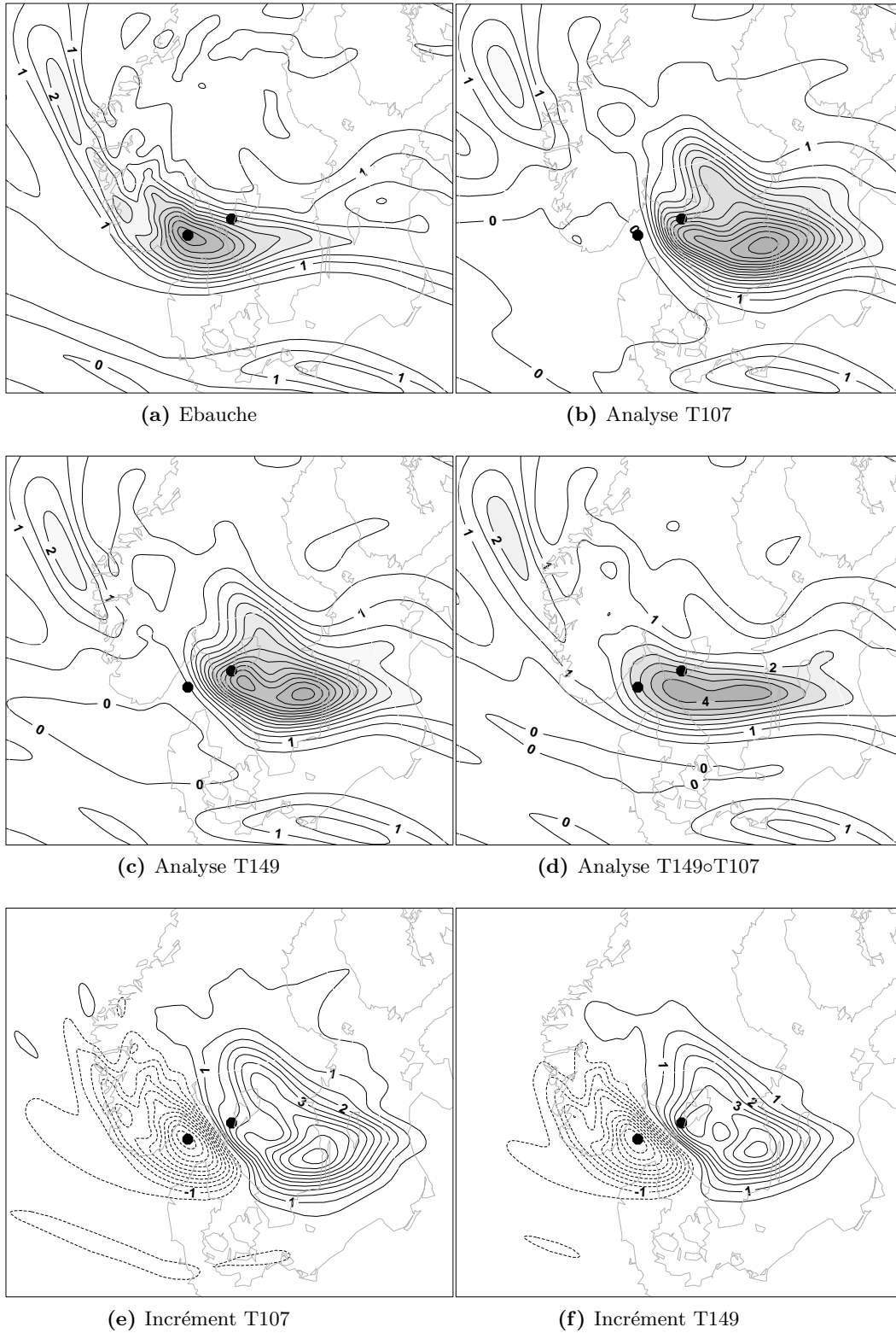
Fig. 4.17: Assimilation à T107, T149 et T149◦T107, cellule 2. Assimilation de pseudo-observations de déplacement pour comparaison des troncutures. Légende identique à celle de la figure 4.16.
