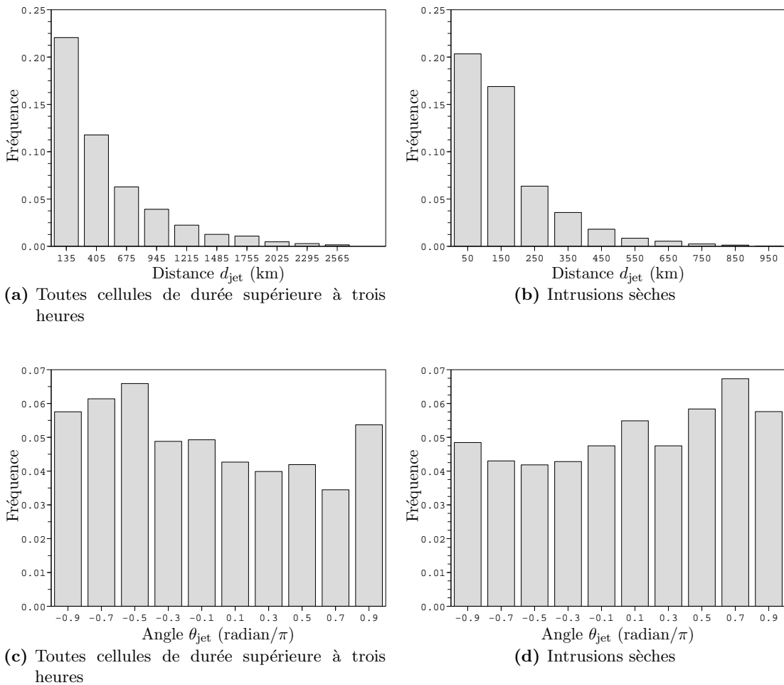
Fig. 1.25: Distributions des distances au jet (en haut) et des angles au jet (en bas) dans l'échantillon d'apprentissage supervisé.
