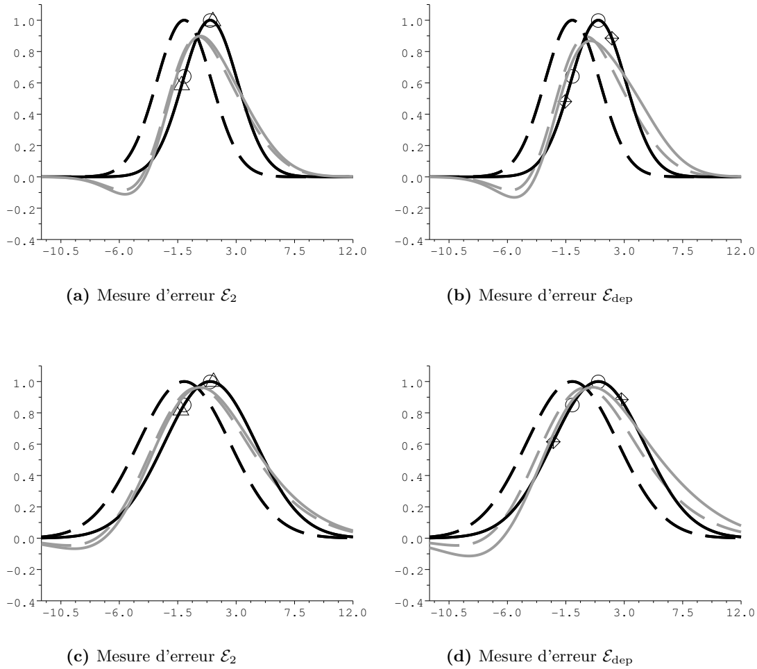
Fig. 4.7: Configurations de pseudo-observations de référence et optimales. En haut, cas où \sigma_o/\sigma_b = 0.3 , L_b/L_a = 4/3 , L_a/\delta_s = 3 . En bas, cas où \sigma_o/\sigma_b = 0.2 , L_b/L_a = 4/3 , L_a/\delta_s = 5 . Légende identique à celle de la figure 4.5.
