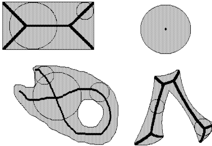
Fig. 1.19: Exemples de squelettes de Lantuéjoul ; figure tirée de Beucher (1990). L'ensemble X est en niveaux de gris, son squelette par boules maximales en traits gras.
