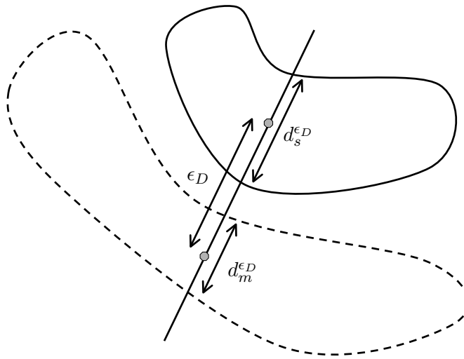
Fig. 4.9: erreur de position \epsilon_D entre cellules modèle et satellite : utilisation des distances caractéristiques d_m^{\epsilon_D} et d_s^{\epsilon_D} dans la direction \epsilon_D .
