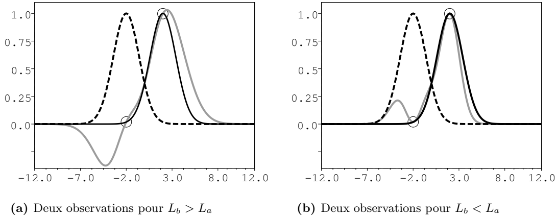
Fig. 4.3: Analyses unidimensionnelles obtenues avec deux pseudo-observations de déplacement de l'ébauche x_b (traits plein à gauche). La pseudo-vérité, ou ébauche déplacée, est en traits plein à droite et sert à générer des observations parfaites (cercles). Les analyses sont en traits tiretés.
