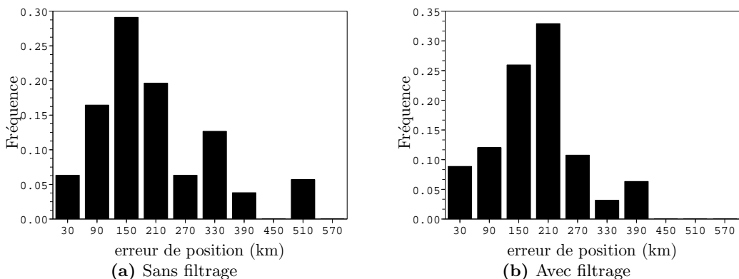
Fig. 4.14: erreur de position mesurée comme la différence des centres de gravité des cellules appariées.
