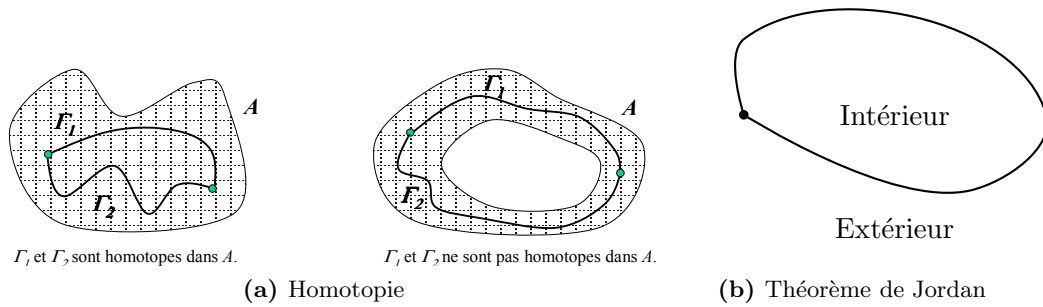
Fig. 1.21: Notion d'homotopie et théorème de Jordan dans \mathbb{R}^2 .
