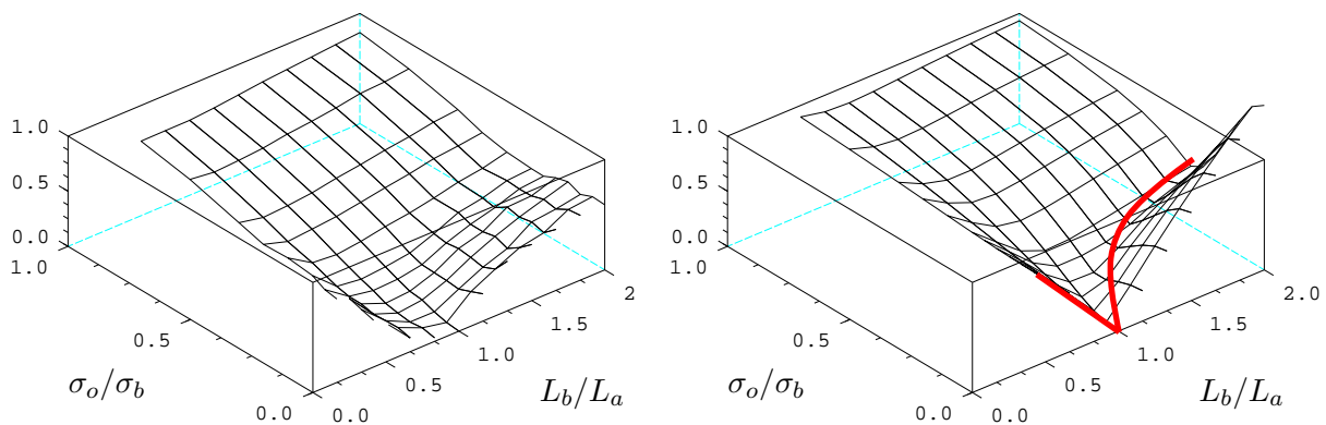
(b) Mesure d'erreur \mathcal{E}_\infty
