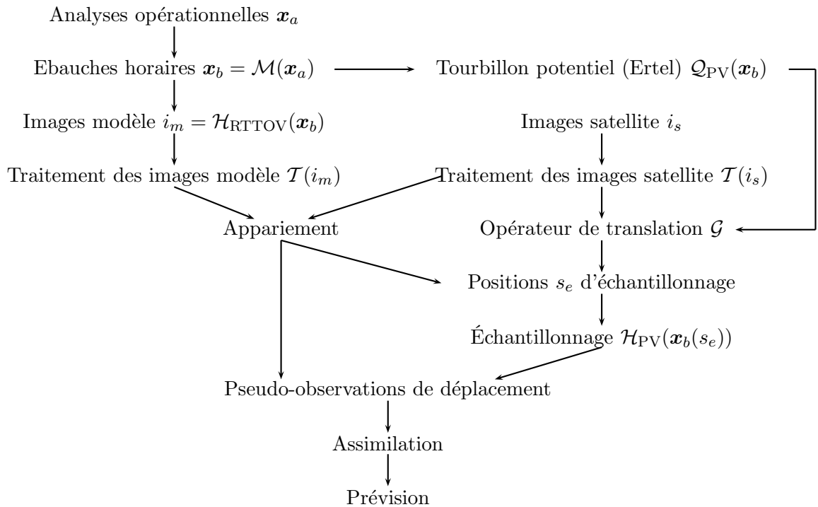
Fig. 4.15: Opérateurs pour la définition et l'assimilation des pseudo-observations de déplacement en tourbillon potentiel d'après les traitements d'images vapeur d'eau.
