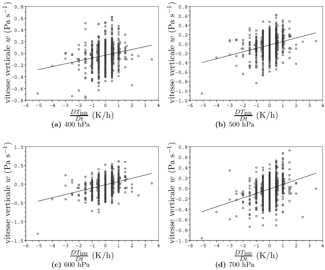
Fig. 3.17: Corrélations entre la vitesse verticale moyennée sur la surface des cellules à un niveau isobare et la variation Lagrangienne de la température de brillance maximale de ces mêmes cellules détectées par Antidote (1570 cas).
