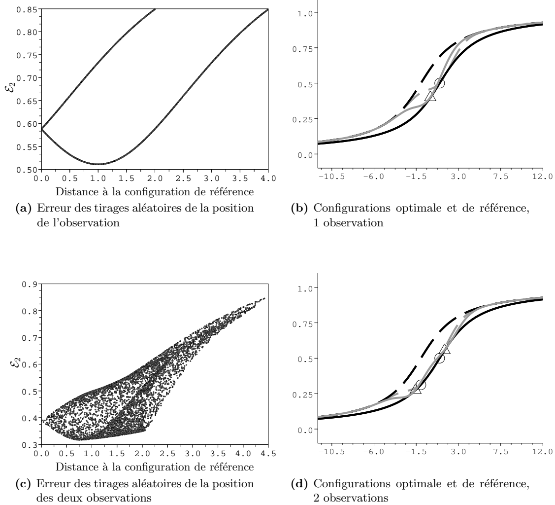
Fig. 4.21: Configurations optimales et de référence pour les pseudo-observations associées au problème de déplacement d'un front. Légende identique à celle de la figure 4.5. Cas où L_b = 2/3 \cdot L_a , \sigma_o = 0.1\sigma_b , L_a/\delta_s = 3 .
