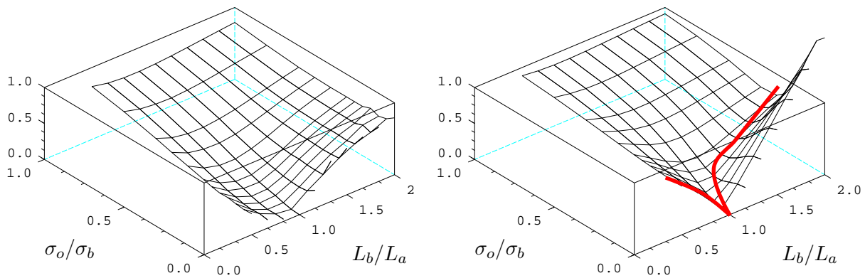
(a) Mesure d'erreur \mathcal{E}_2
