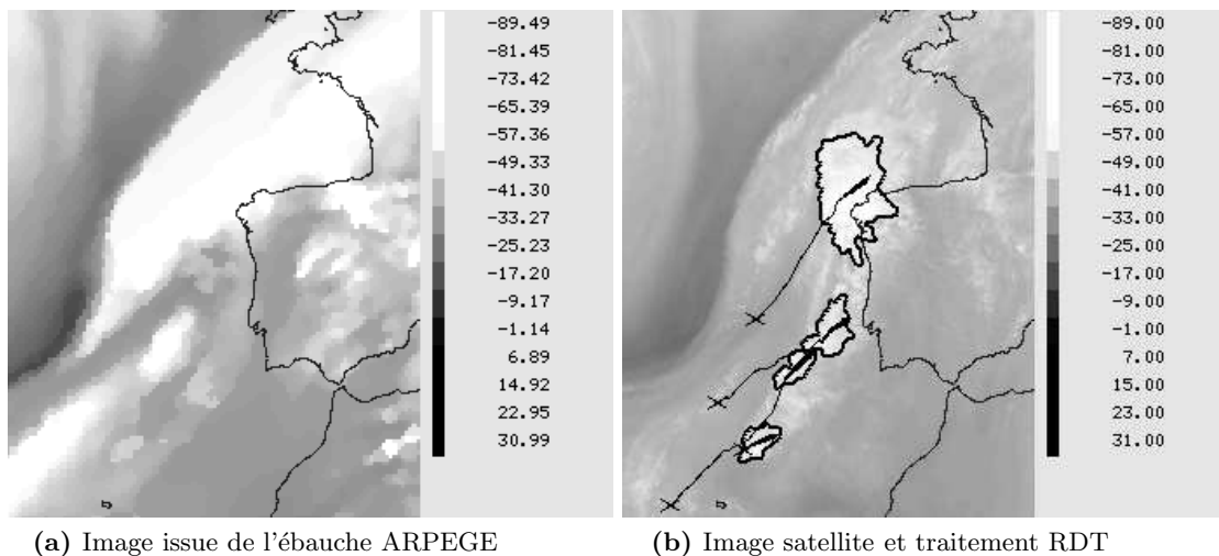
Fig. 6.3: Image satellite modèle valide au 02/10/2006 12 TU issue d'une ébauche ARPEGE (prévision à six heure, panneau de gauche). Suivi des systèmes convectifs de mésoéchelle dans l'imagerie vapeur d'eau, à la même date (à droite).
