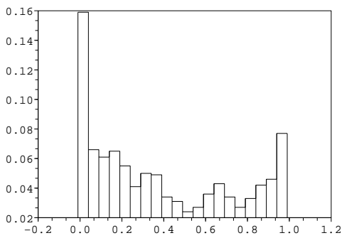
(c) Histogramme des erreurs en s = 0
