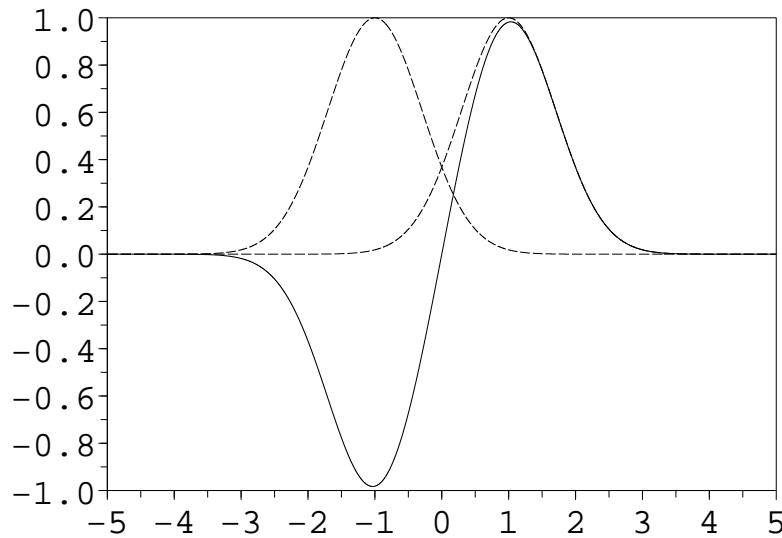
Fig. 4.2: Incrément d'analyse pour des fonctions de structures gaussiennes homogènes et une innovation symétrique. Les observations sont en s = \pm 1 .
