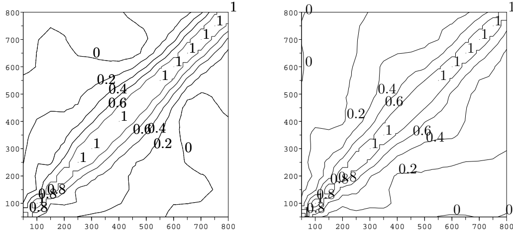
(a) Matrice de corrélation associée à B
