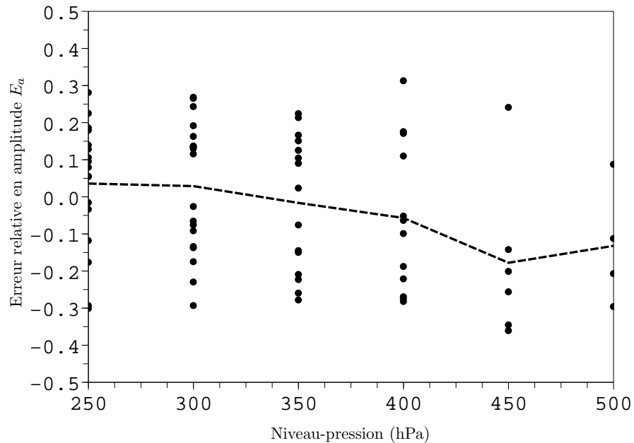
(a) Erreur relative d'amplitude
