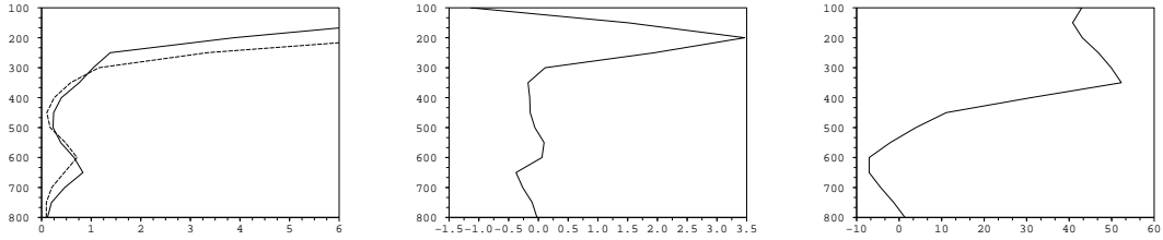
(a) Profils de PV distant de six heures (b) Différence en amplitude (PVU) (c) Différence en position (hPa)
