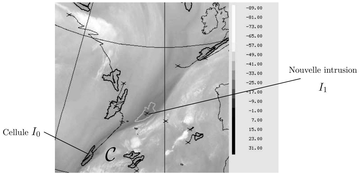
(b) Suivi non filtré au 02 Octobre 2006 à 01h45 TU - zoom en 32N, 25W
