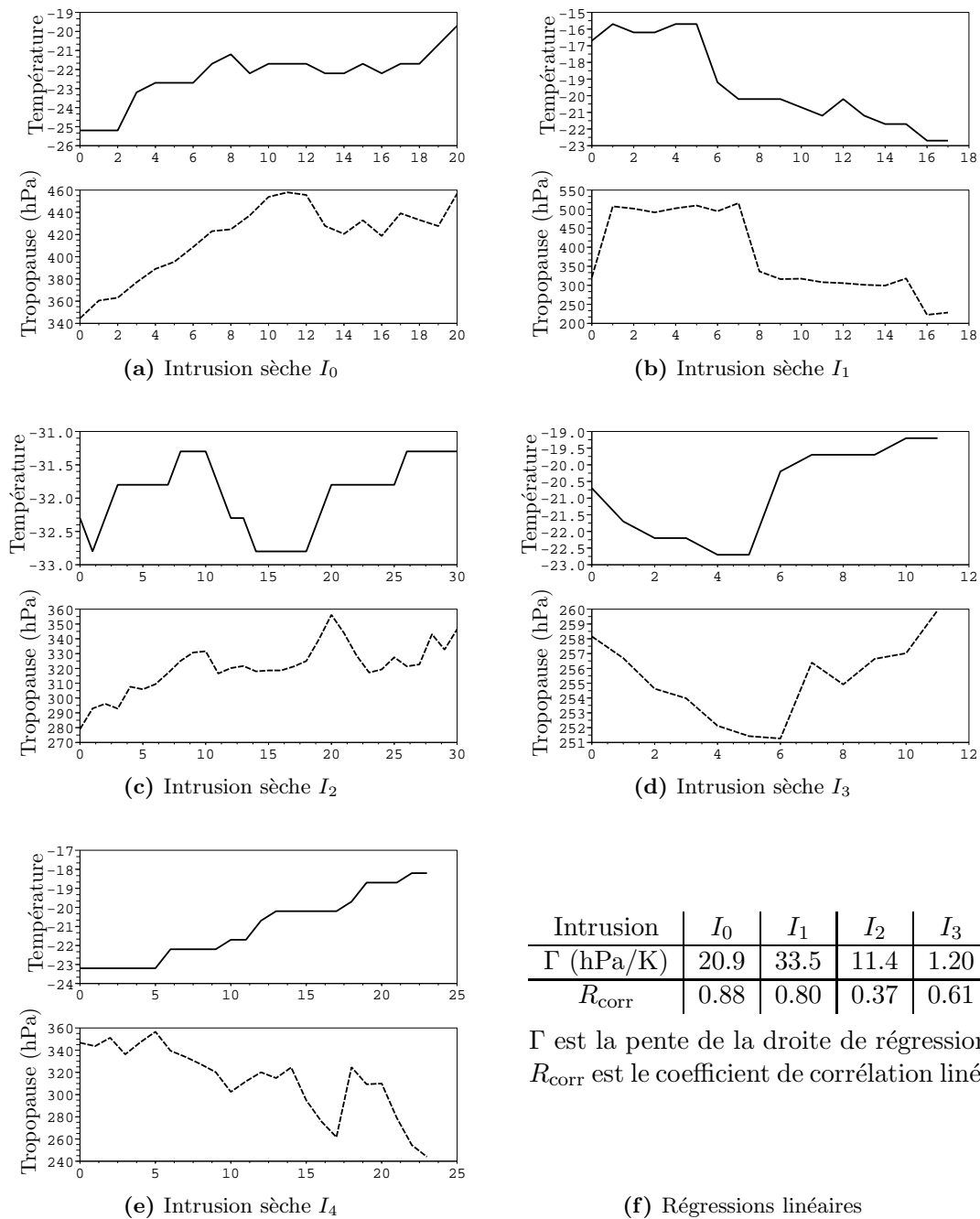
Fig. 6.6: Évolutions temporelles comparées de la température de brillance et de la hauteur moyenne de la tropopause pour différentes trajectoires d'intrusions sèches détectées sur les images modèle.
