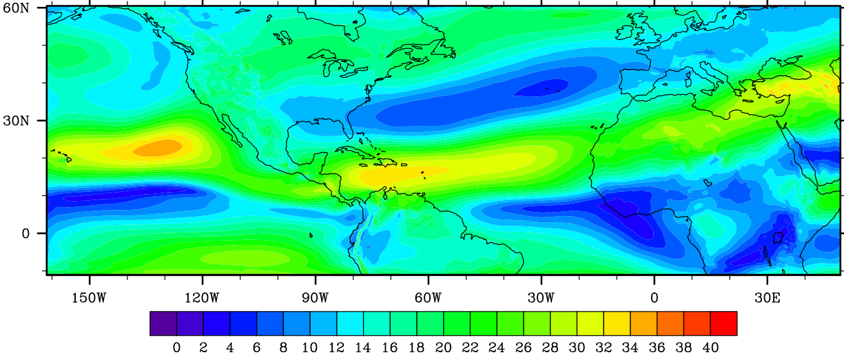
dudz ASO ave dom1_ens1_19952005
