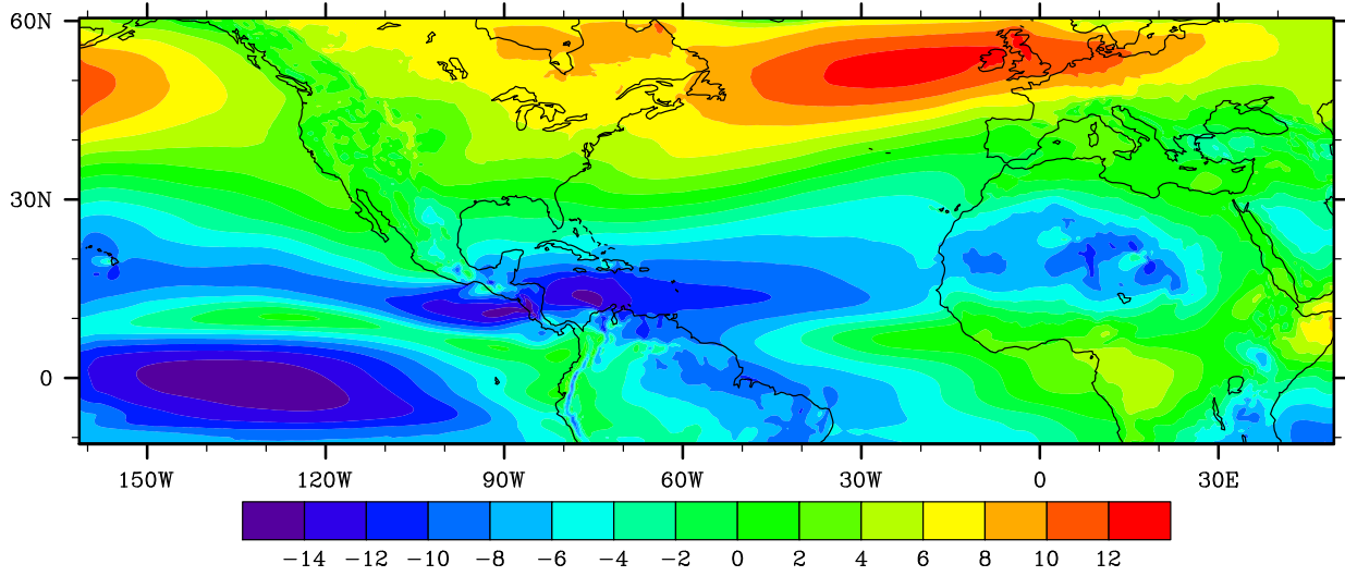
U 850mb ASO ave dom1_ens1_19952005
