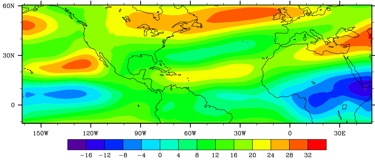
U 200mb ASO ave dom1_ens1_19952005
