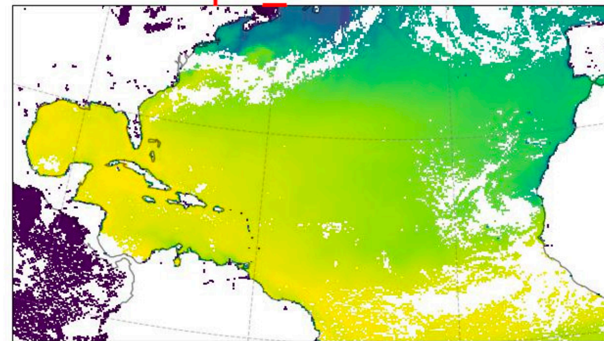
oops_nomask
